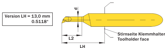
Abbildung zeigt / Drawing shows: A05.2025.20.52.20 Y R
